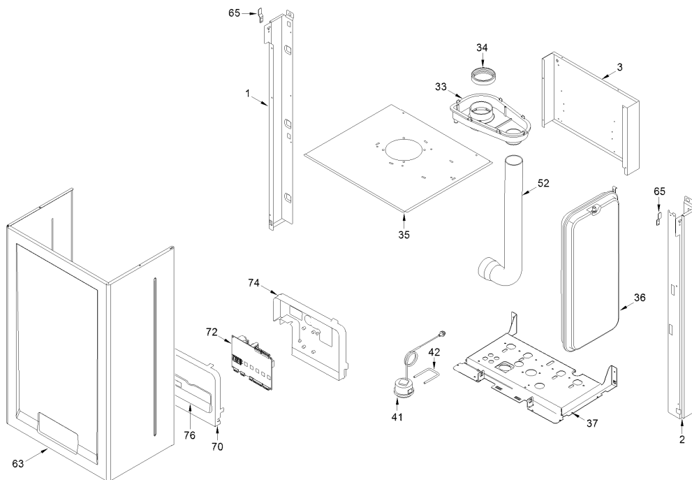
BRAVA DGT HE 35 - telaio / pannello strumenti
